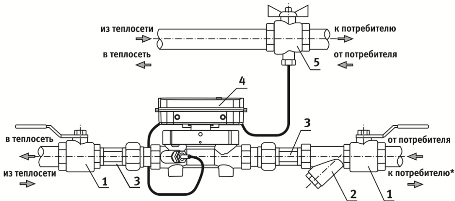
1 - кран шаровый; 2 - фильтр сетчатый муфтовый; 3 – муфта соединительная; 4 – теплосчетчик с интегрированным ПР и ТС; 5 – кран шаровый для монтажа ТС.
