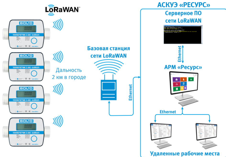
Рисунок №2. Схема построения сети LoRaWAN
